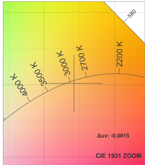
CRI: 81,1 (R1-R8)
