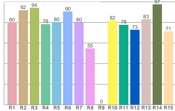
CRI: 81,1 (R1-R8)
