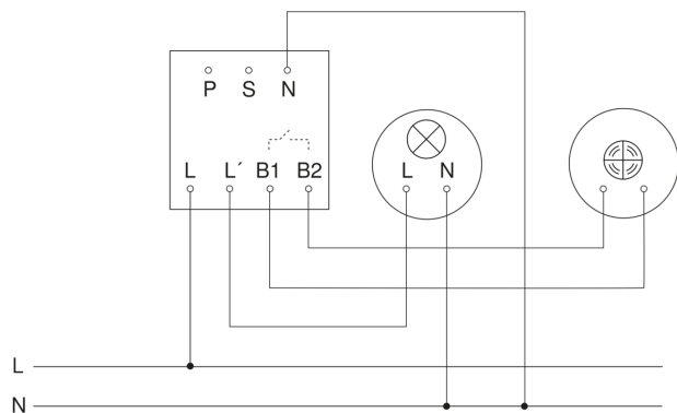
Schaltplan Master
